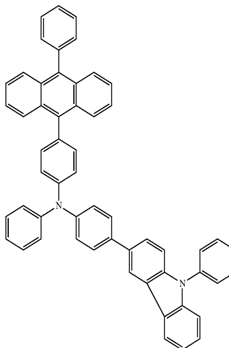
PCBAPA
