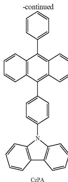
CzPA
