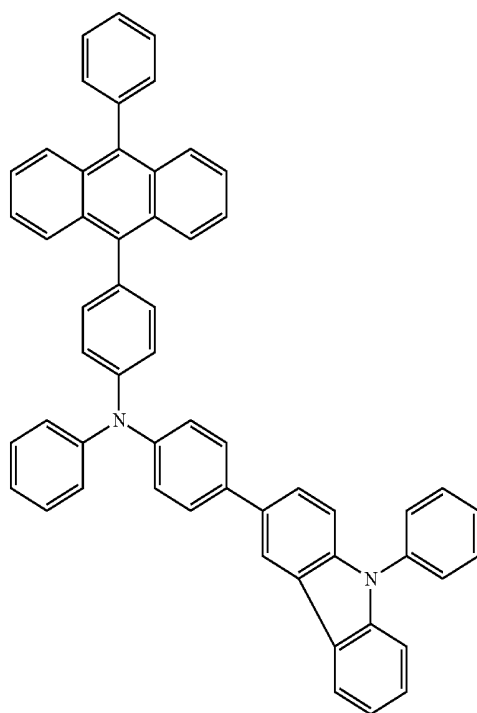
PCBAPA
